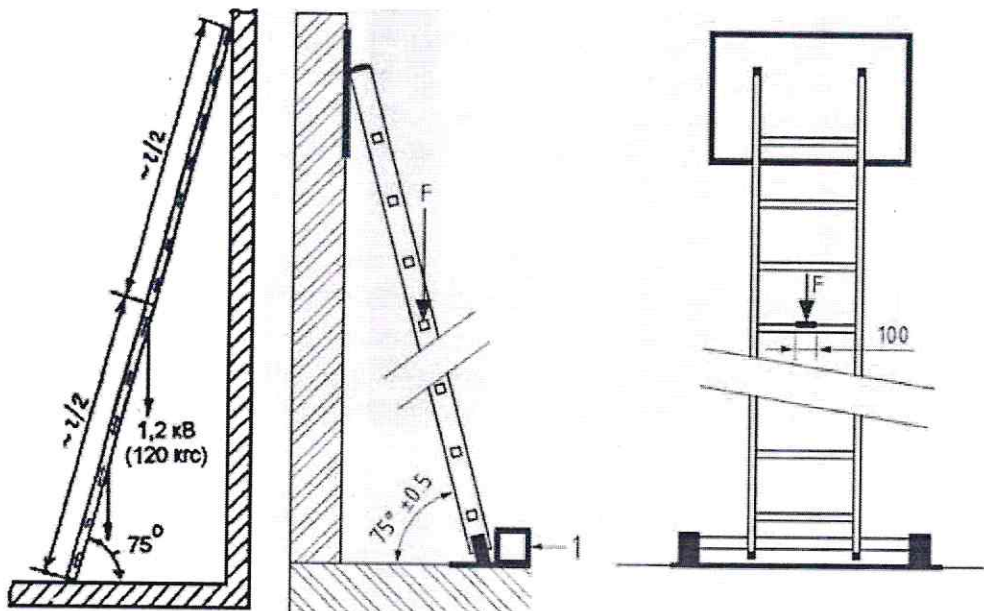
Рис.1. Схема испытания приставной лестницы
